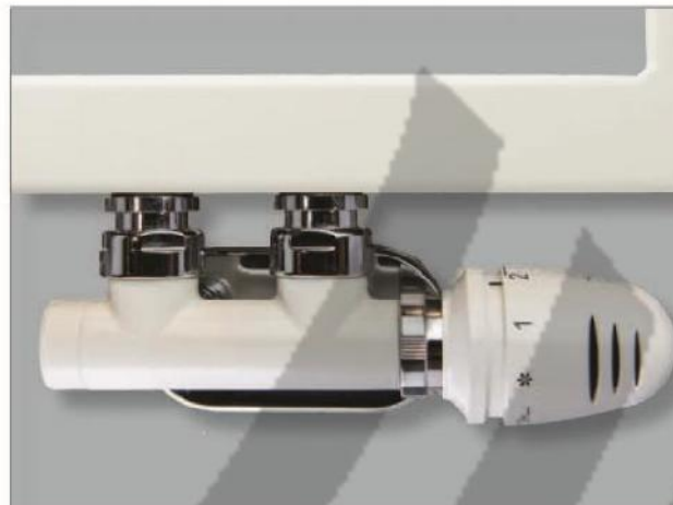
Cap termostatic MINI DE LUXE, alb Garnitură robinet termostatic TS-3000 E bitubular, alb Conector 16*2 mm (2 buc.) Set piese de mascare țevă
