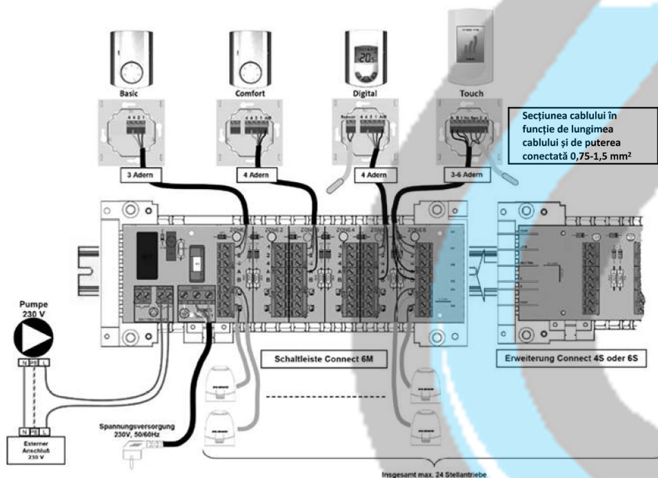
Figura 122 TempCo Cool 230 V
